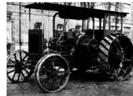
Колесный трактор с керосиновым двигателем производства Коломенского машиностроительного завода. 1917 год
