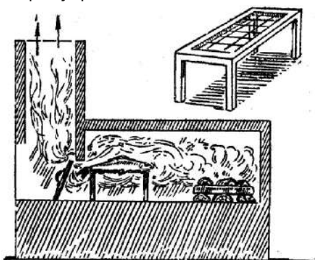
Рис. 10. Схема горячего копчения рыбы в русской печи (сверху показана подставка для рыбы)
