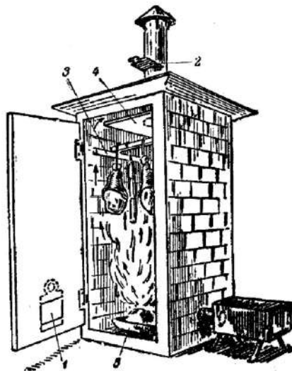
Рис. 9. Домашняя коптильня: 1 и 2 - задвижки для регулирования доступа воздуха и выхода дыма; 3 - поперечные перекладины для укрепления на них палок (вешал); 4 - железный лист; 5 - железный поддон с тлеющими опилками; 6 - печка, присоединенная к коптильне
